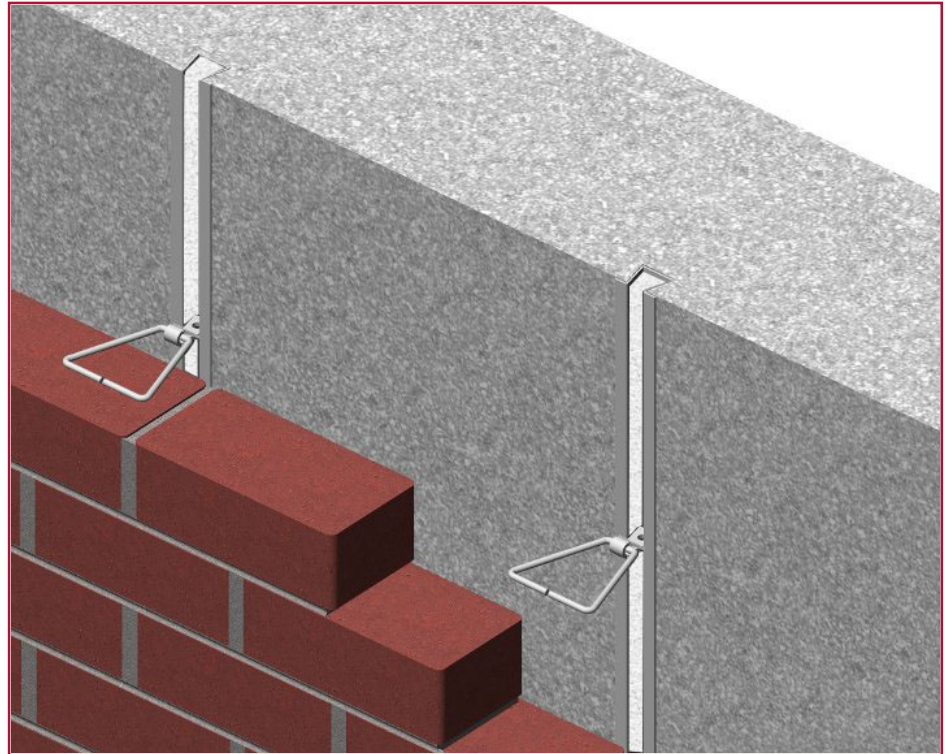
↑ # 1304 Dovetail Slot
